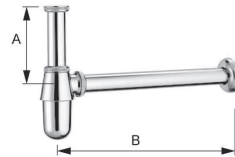
Bottle-Trap 6512-BT-80CP A:108 B:210 mm 6512-BT-81CP A:108 B:420 mm 6512-BL-80CP A:185 B:210 mm 6512-BL-81CP A:185 B:420 mm
