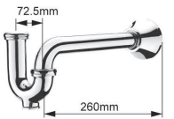
P-Trap W/Cleanout 6119-A3-80CP 1 1/2" 6119-B3-80CP 1 1/4"
