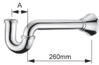
P-Trap 6122-A3-80CP A:73mm 1 1/2" 6122-B3-80CP A:65mm 1 1/4"
